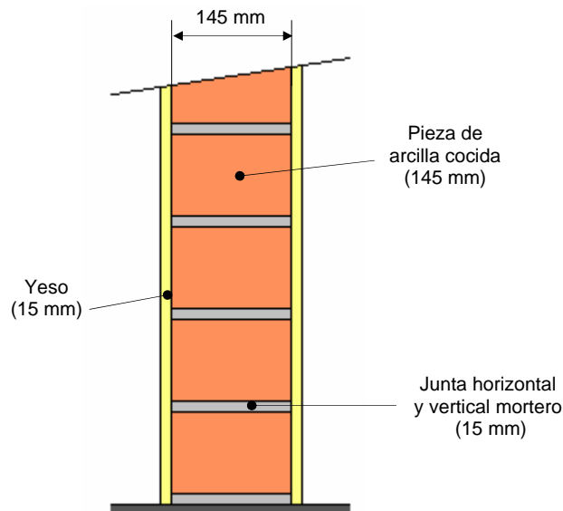
Figura 1: Esquema de muestra ensayada (B2012-22-M36)
