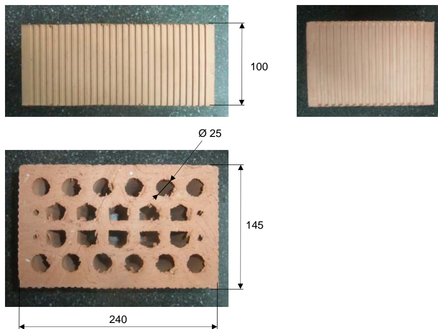
Figura 2: Dimensiones medidas de pieza de arcilla cocida (cotas en mm)
